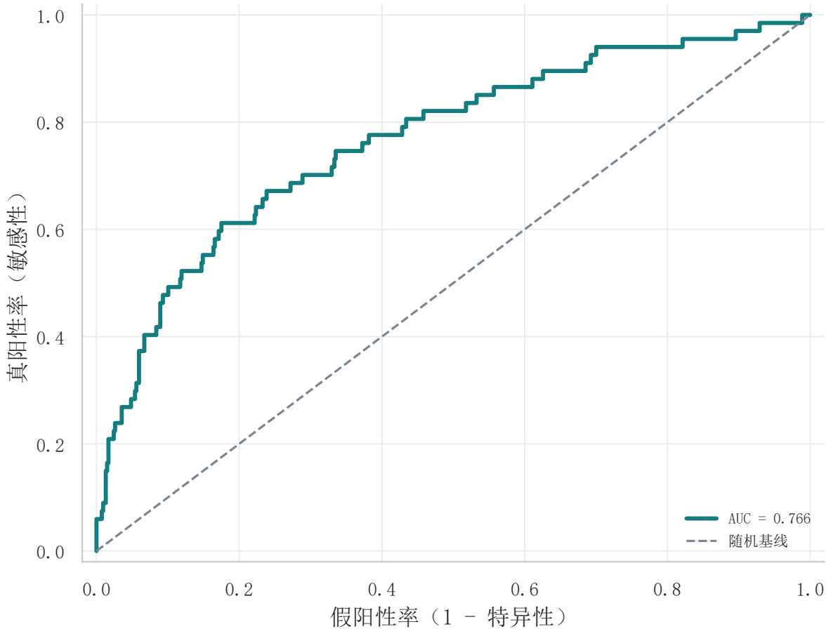
Q4 Elastic-Net 分类器 ROC (AUC=0.766)
