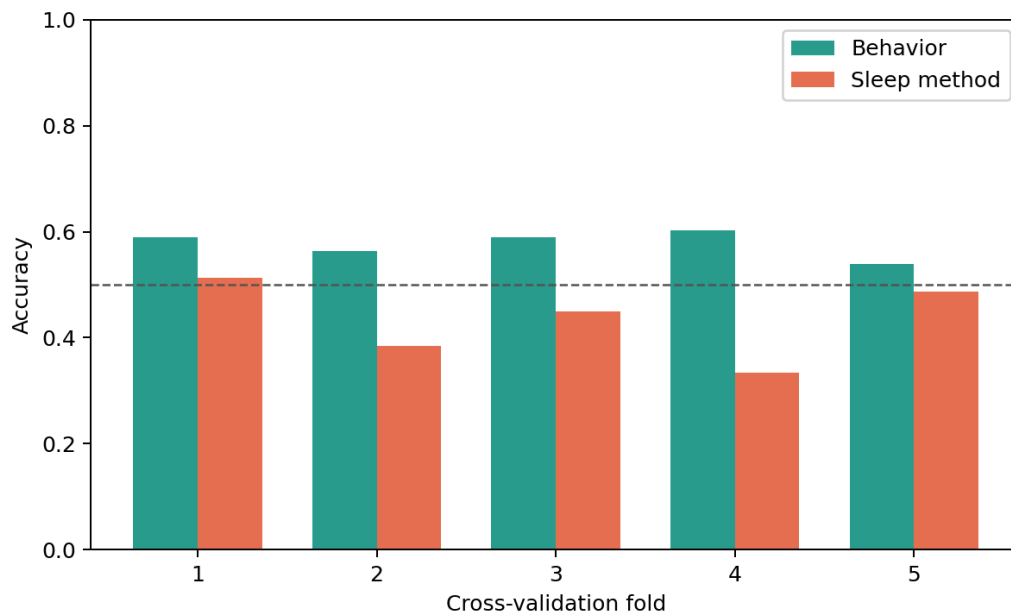
Figure 2: 行为与入睡方式的逐折准确率。
