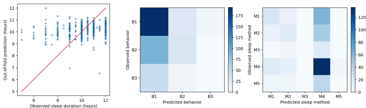
Figure 1: 睡眠时长样本外预测以及行为、入睡方式混淆矩阵。
