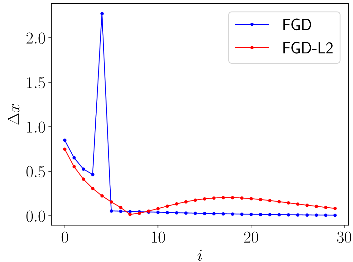
(d) Trajectory of \Delta x at \alpha = 0.5
