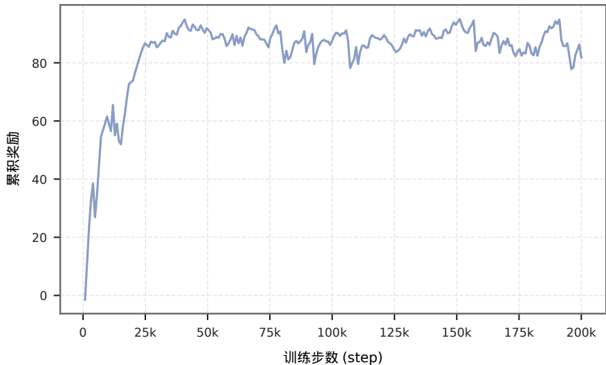
训练过程累积奖励曲线
