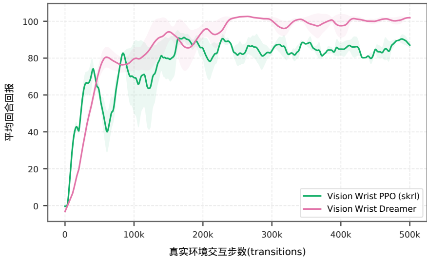
平均回合回报
