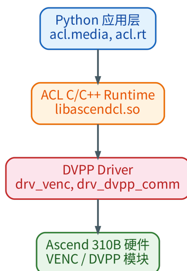
Figure 5.1.: CANN/ACL 与 DVPP 的调用层次
