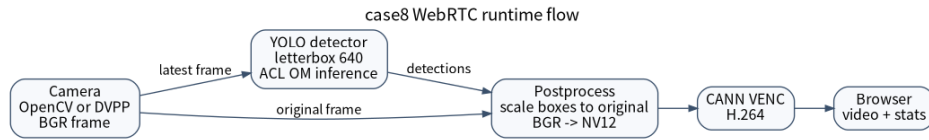
图 3：case8 WebRTC 流水线。
