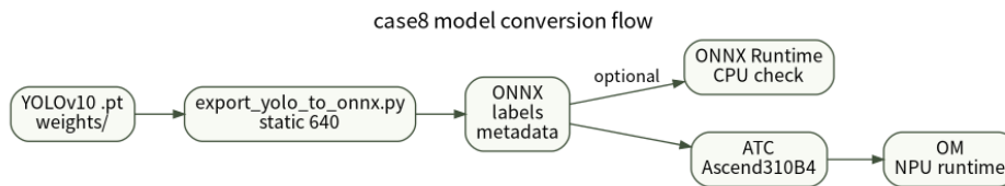
图 2：case8 模型转换流程。
