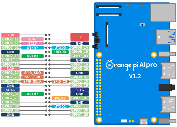
Figure 4.: GPIO 接口定义
