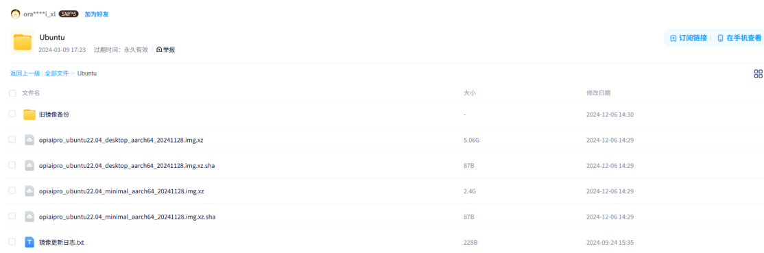
Figure 26.: 选择镜像
