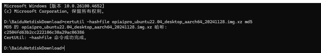
Figure 28.: md5 校验
