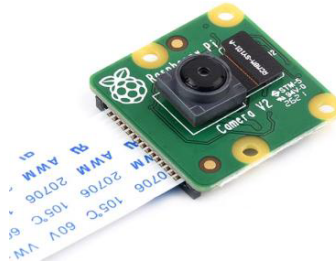
Figure 18.: MIPI-CSI 摄像头
