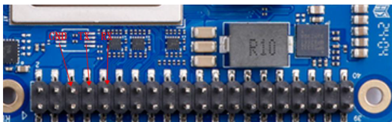
Figure 43.: 开发板串口
