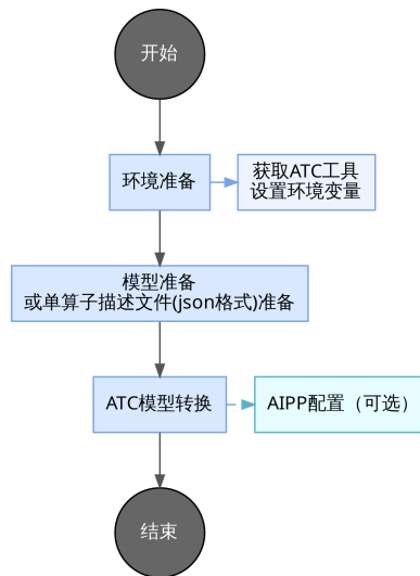
Figure 2.4.: ATC 流程图
