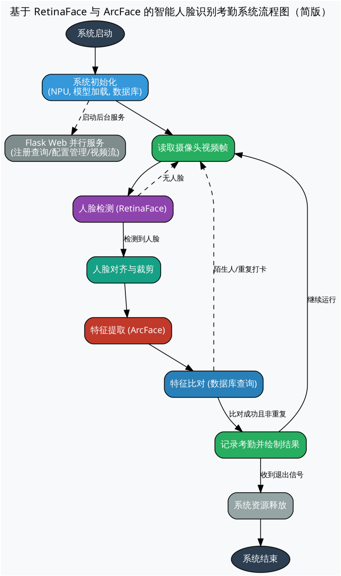
Figure 1.1.: 程序流程图
