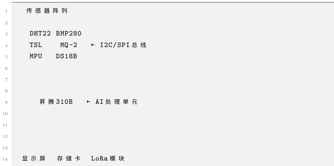
系统架构图
