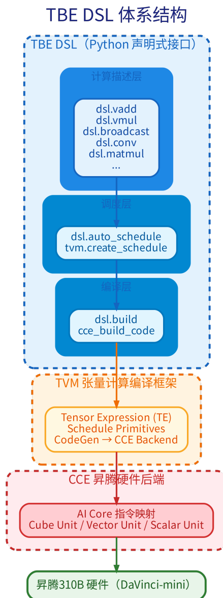
Figure 6.1.: TBE DSL 体系结构
