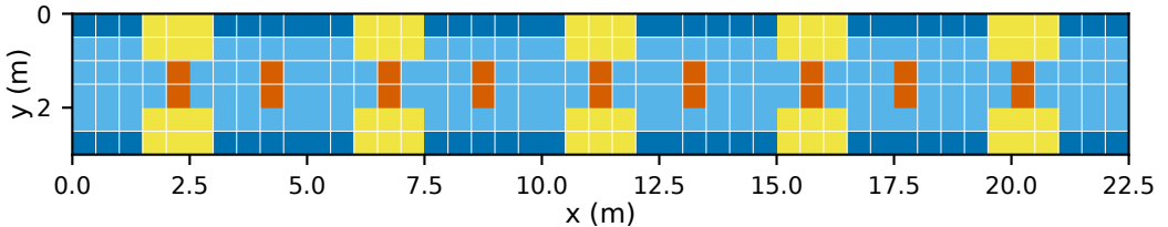
(d) Metro carriage: 45×6, a = 0.5 m, N = 310
