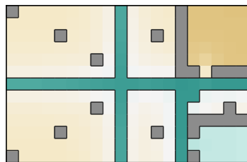
(a) 平均场
