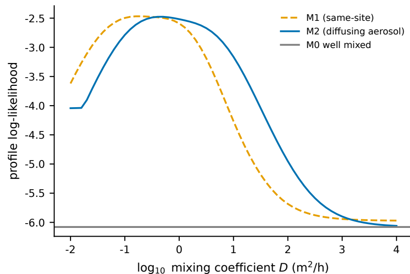
(d) Guangzhou restaurant: likelihood of D
