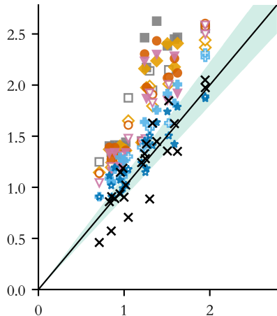
首例的二代病例数 (实测接触)
