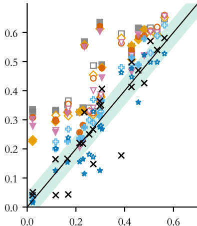
发生大规模暴发的概率 (实测接触)
