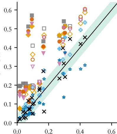
平均罹患率 (实测接触)
