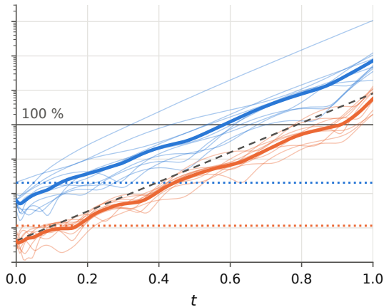
(b) Sobol'
