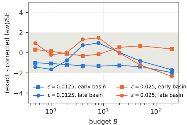
(d) residuals; limit law: up to 43.1 SE
