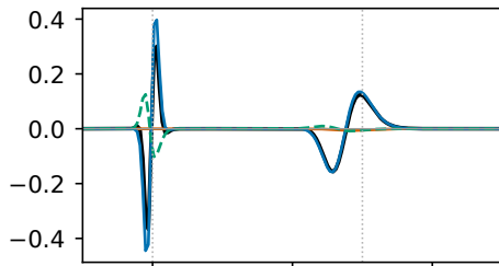
(d) m = 3, \varepsilon = 0.1, B = 4
