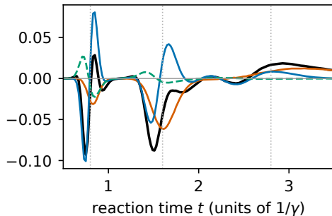
(d) m = 3, \varepsilon = 0.1, B = 4
