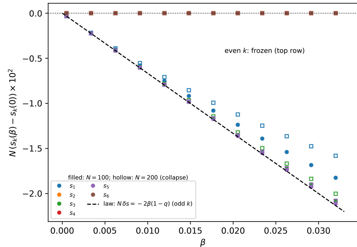
(2) the roots move TRIVIAIY ( N -collapse)
