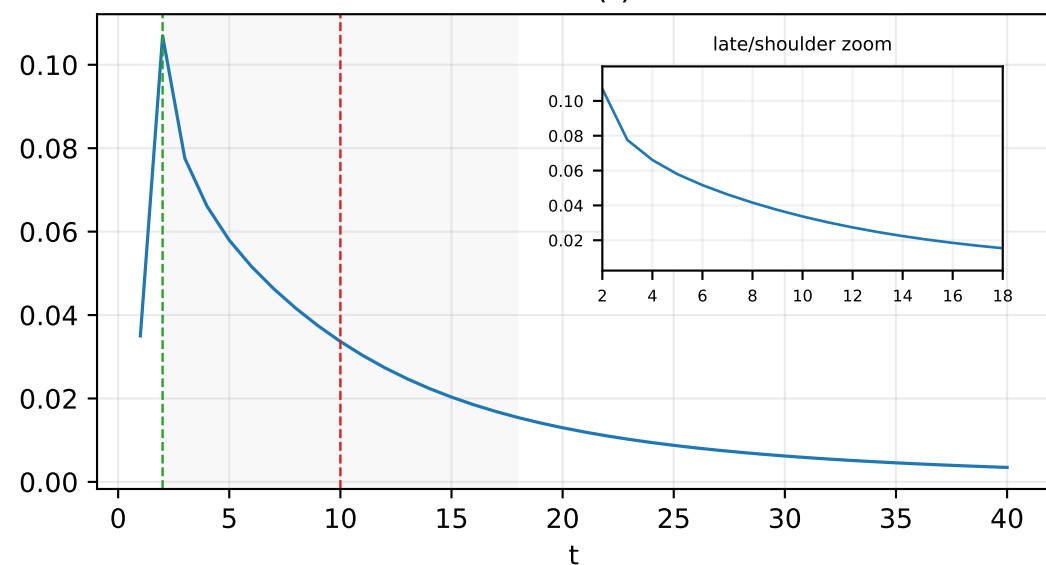
F2=f(2n-1)+f(2n)
