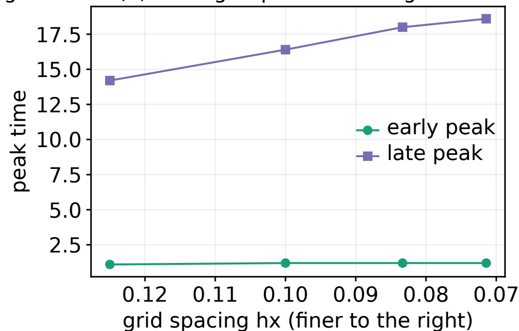
(d) finite-grid peak-time diagnostic
