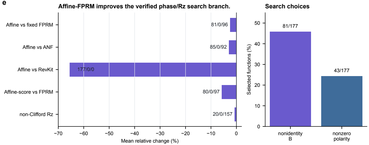
图 6: Affine-FPRM 相位搜索。左图为 Affine-FPRM 相对 fixed FPRM、ANF 和 RevKit proxy 的平均变化；右图为非 identity 线性变换和非零极性的选择频率；源数据见 fig4_phase_affine.csv 。
