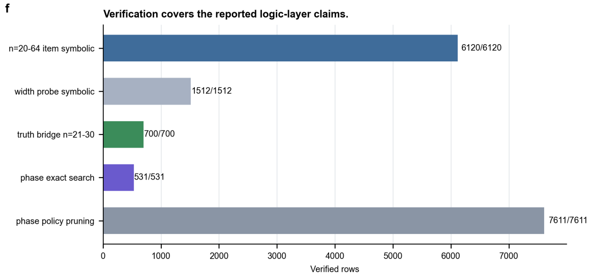
图 7: 验证覆盖。主图区分符号验证、phase/policy 验证和完整 真值表 bridge; 不同验证强度不作等价解释。Source data: fig5_validation.csv.
