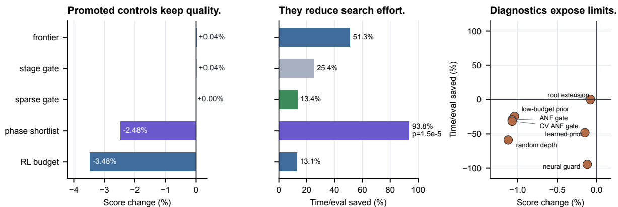
图 5: 学习与搜索控制证据汇总。promoted controls 同时具备可验证的质量或开销收益；limited diagnostics 则保留小幅质量、运行时间反向或代理边界，防止把所有 AI 模块写成同等主贡献。Source data: fig7_learned_control_summary.csv.
