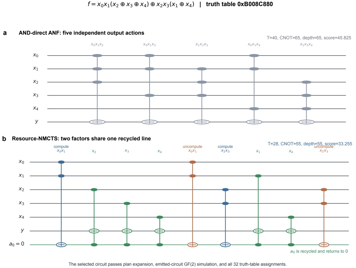
图 2: Resource-NMCTS 的完整线路实例。(a) AND-direct ANF 对式 (5) 中每个单项式施加独立三控操作; (b) Resource-NMCTS 按式 (6) 执行 compute/reuse/uncompute, 并把复用辅助线恢复为 0。图中是通过验证的 X/CNOT/MCT 逻辑骨架; 资源数字采用本文 logical-AND 口径, 其中合取计算使用 4T, 反计算使用 Clifford/measurement-assisted accounting。Source data: fig8_worked_example.csv.
