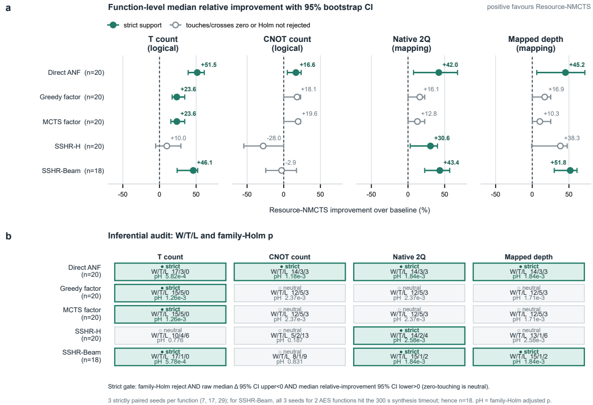
图 5: 冻结主结果与推断审计。 a Resource-NMCTS 相对五个基线的函数级中位相对改善及 95% bootstrap CI, 正值有利; 实心绿色仅标记同时通过双区间与分族 Holm 门槛的比较。 b 每格给出独立函数数、胜/平/负和分族 Holm 校正 p_H 。每个函数先严格配对 seed 7/17/29; SSHR-Beam 的两个 AES 函数均达到 300 s 综合超时, 故该比较 n = 18 。Source data are provided in the figure source CSV/JSON.
