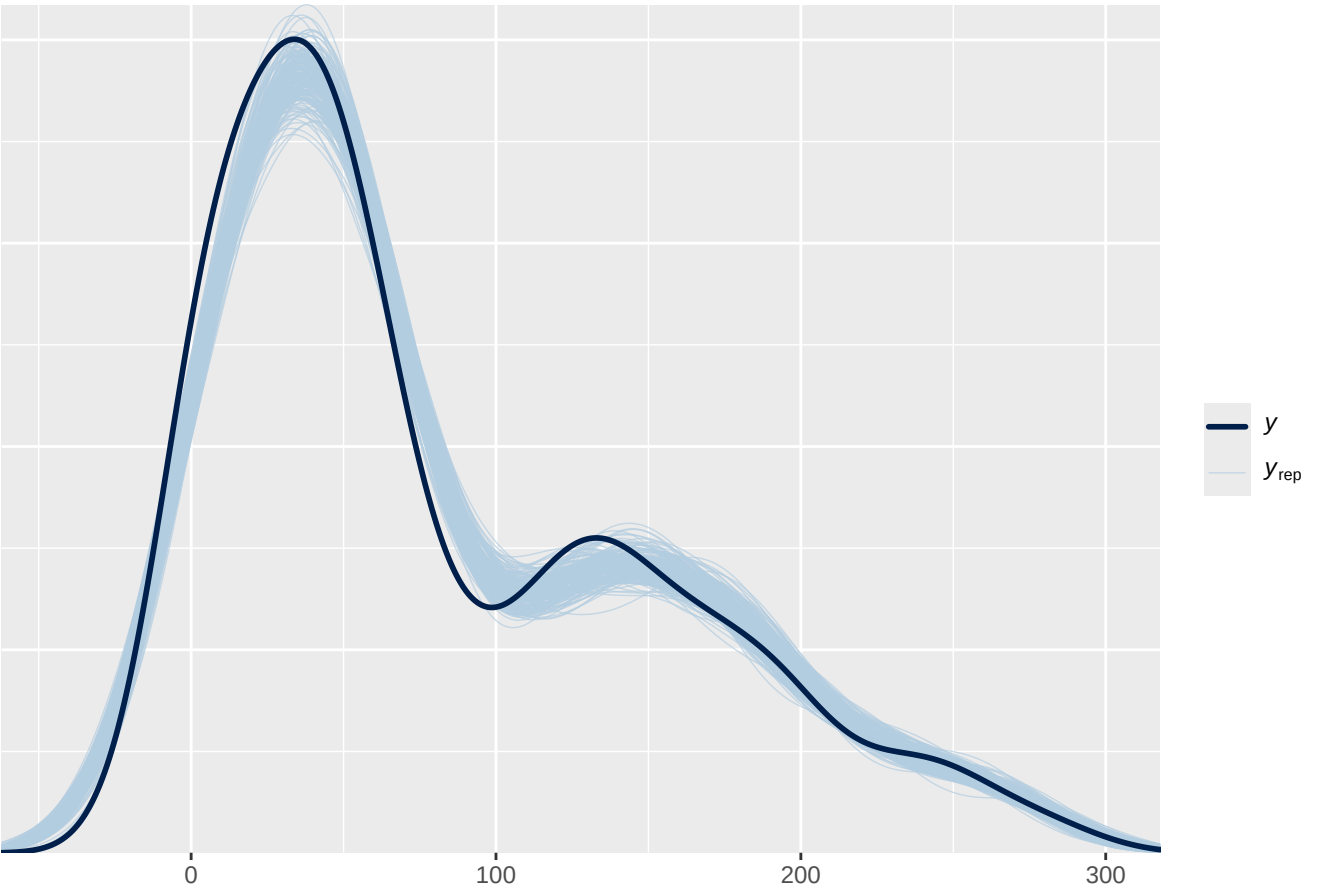
PPC density overlay: vanLeeuwen_q
