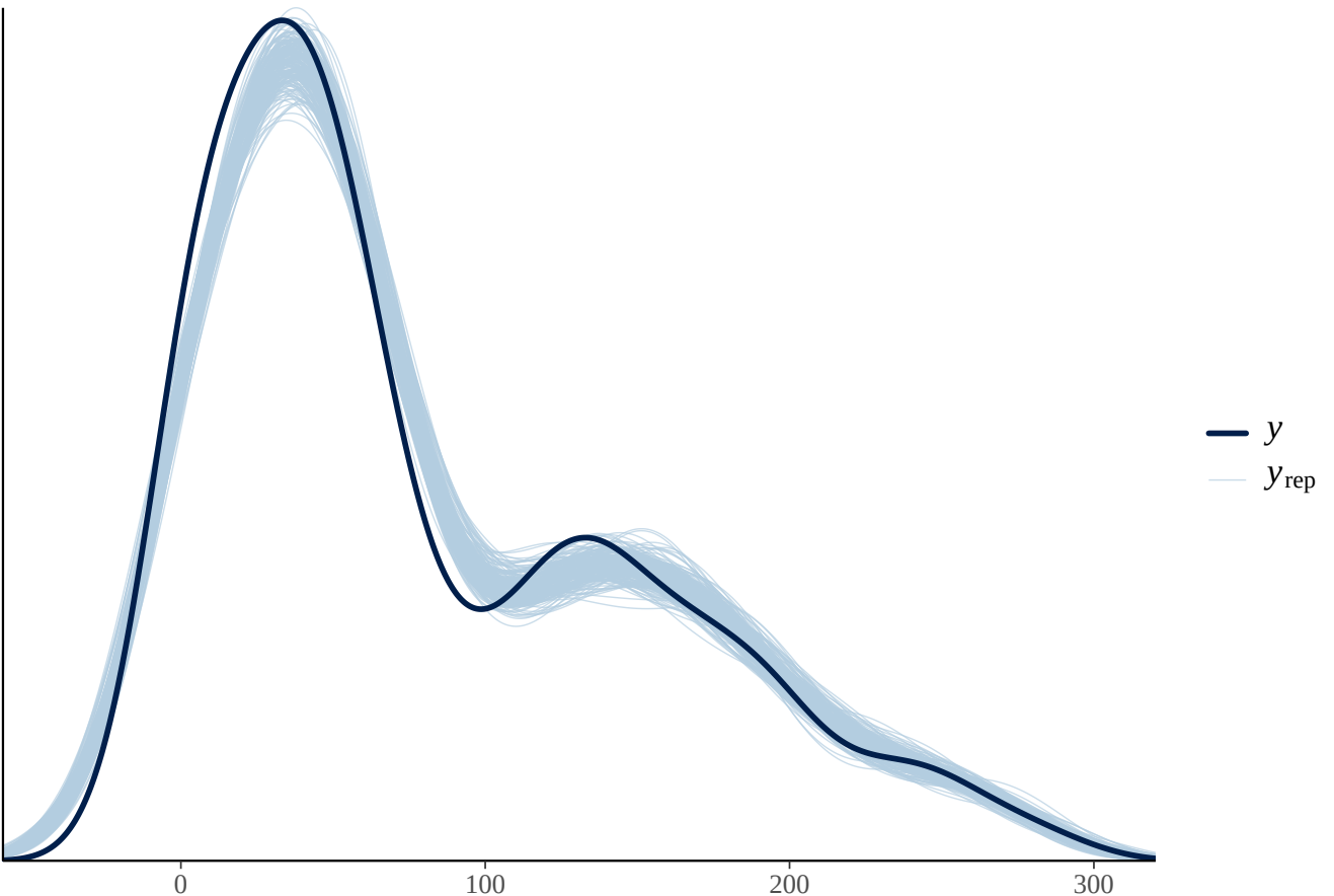
PPC density overlay: vanLeeuwen_z
