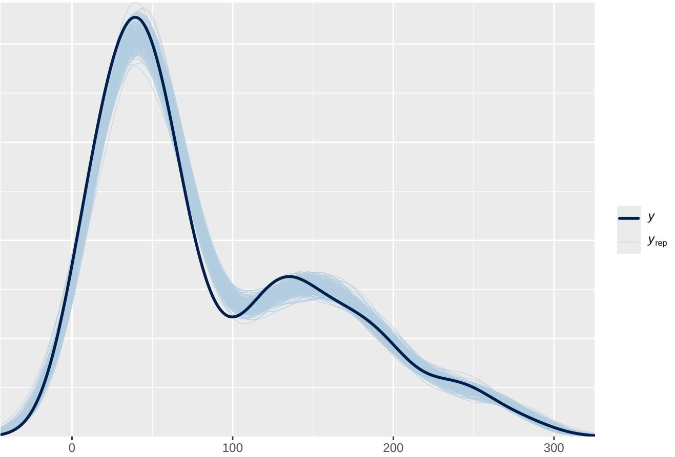
PPC density overlay: vanLeeuwen_wq
