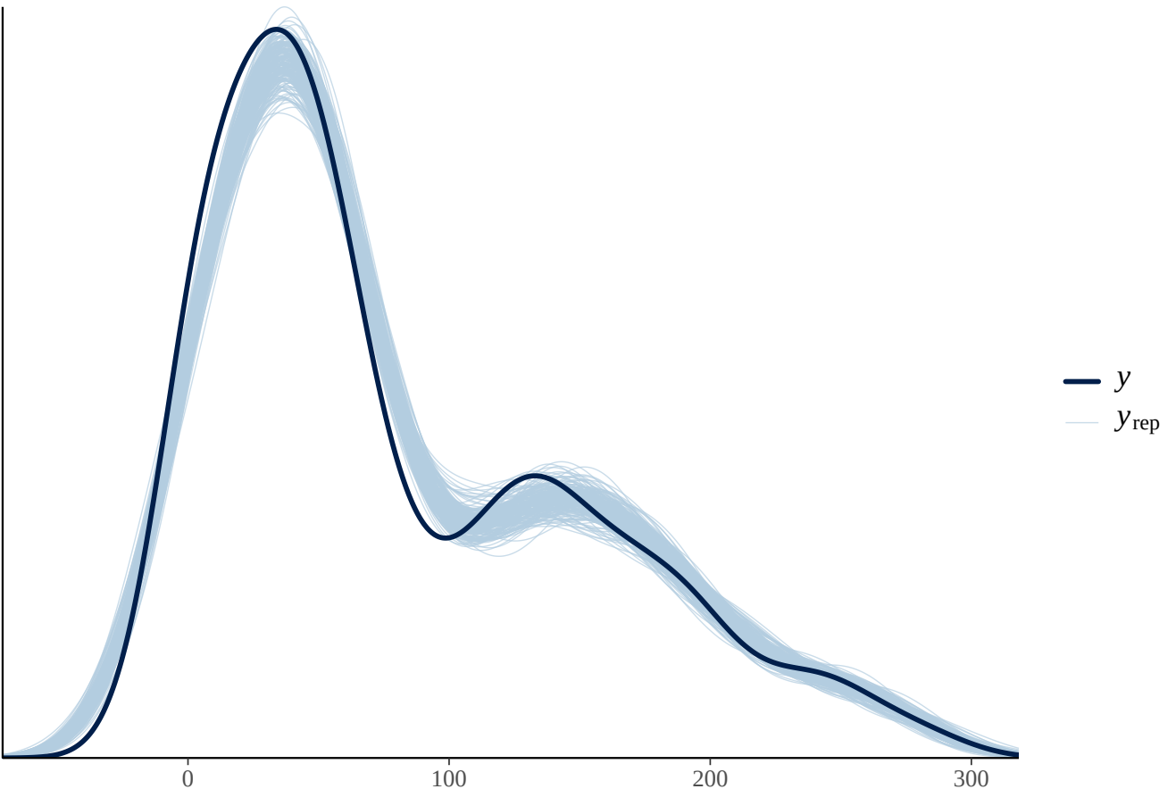
PPC density overlay: vanLeeuwen
