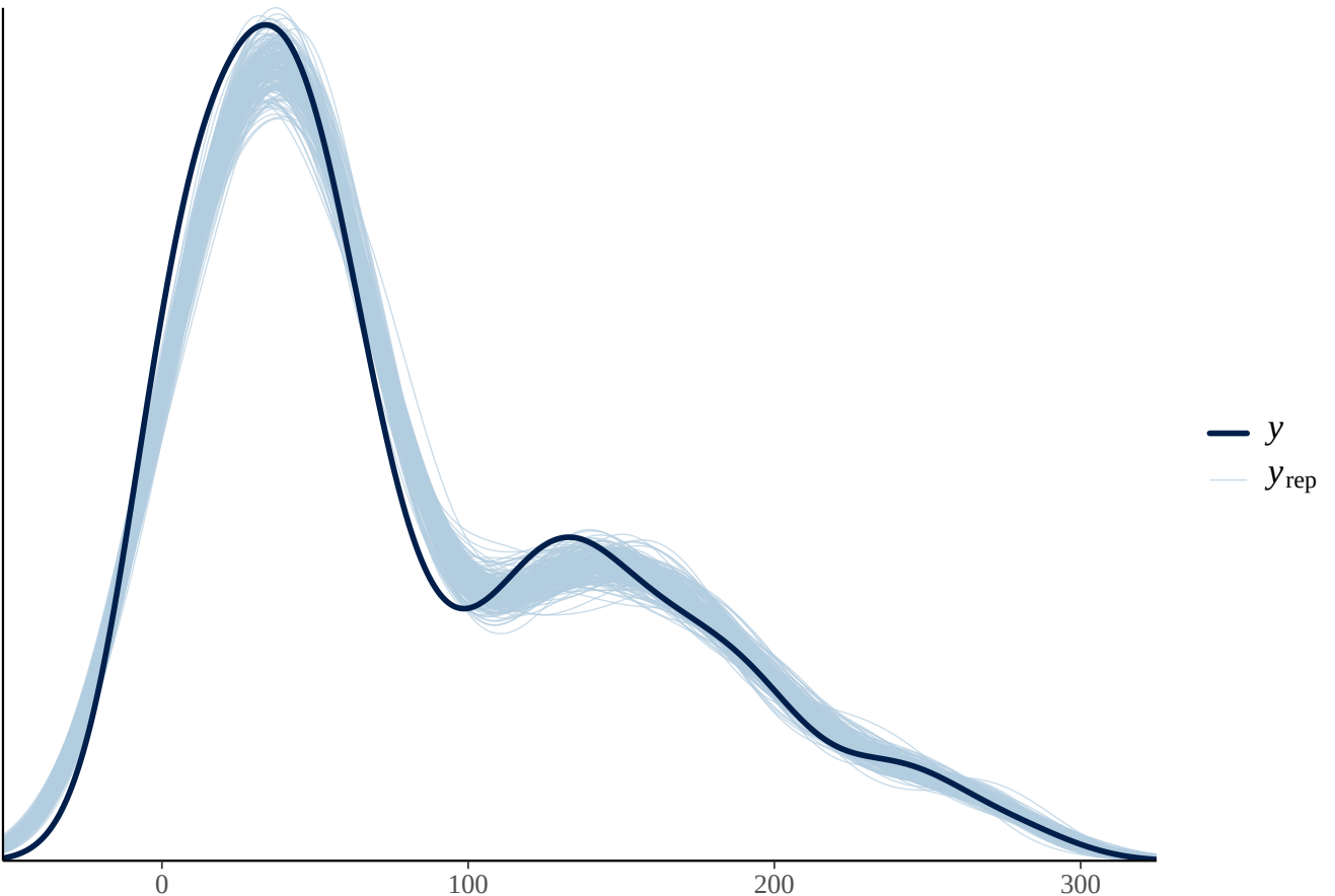
PPC density overlay: vanLeeuwen_q_z
