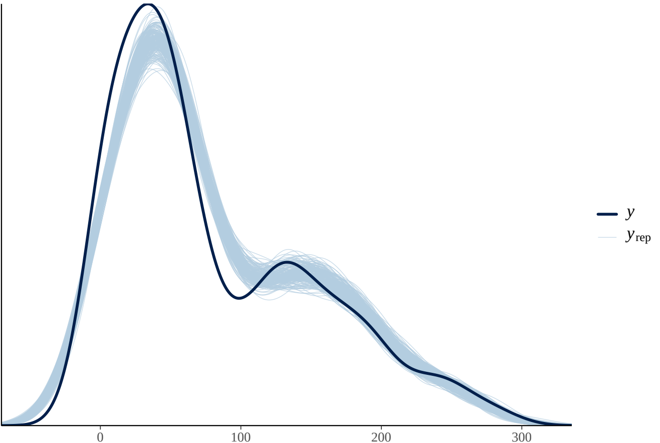
PPC density overlay: vanLeeuwen_z_noM
