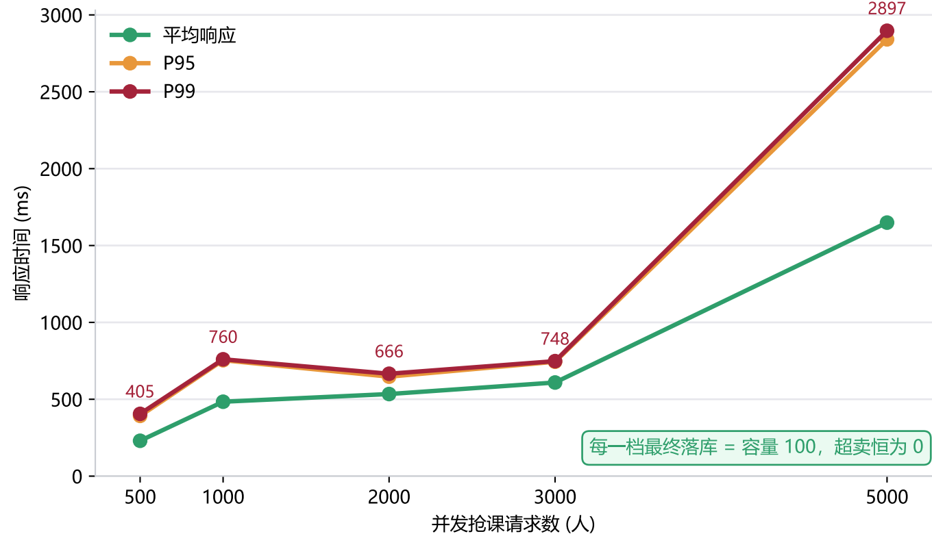
不同并发下的响应时间 (容量=100, 每档 3 遍取中位)
