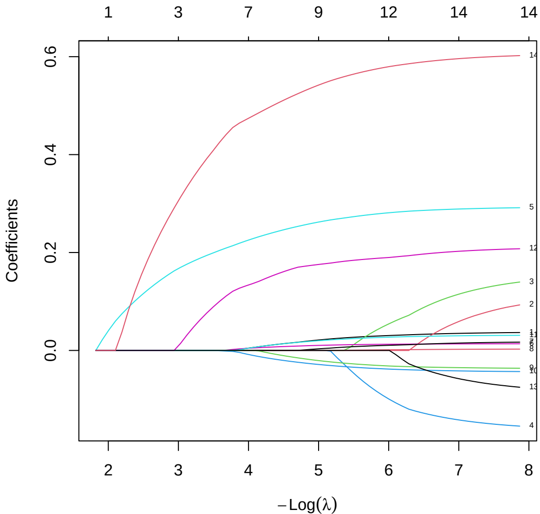
A: LASSO Coefficient Paths
