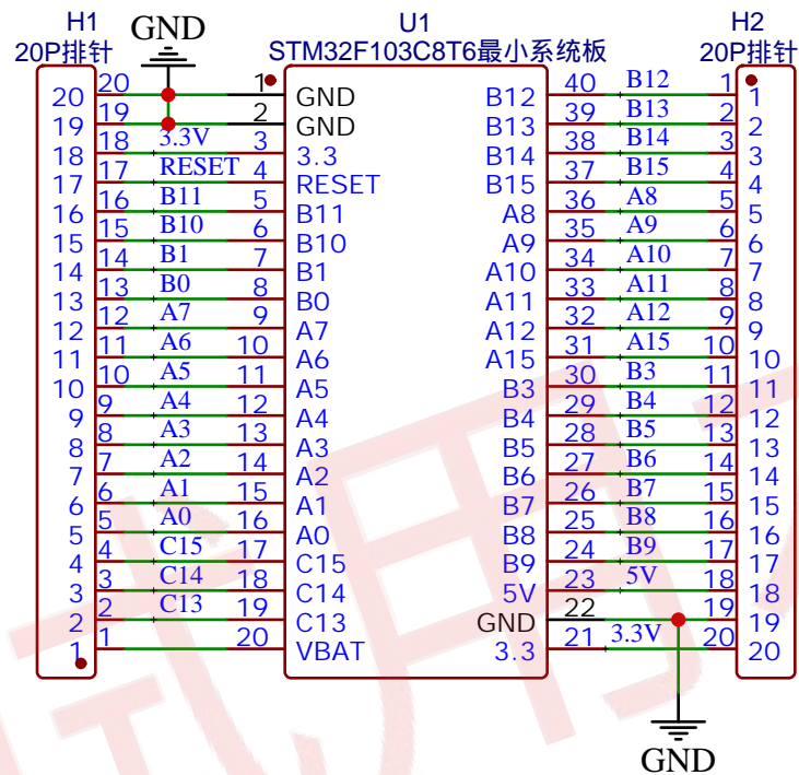
主控STM32F103C8T6
