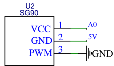
SG90舵机
