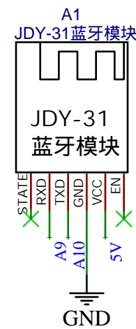
蓝牙模块
