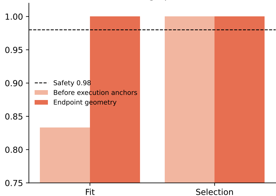
Verified edge precision
