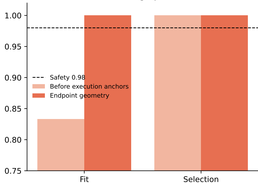
Verified edge precision
