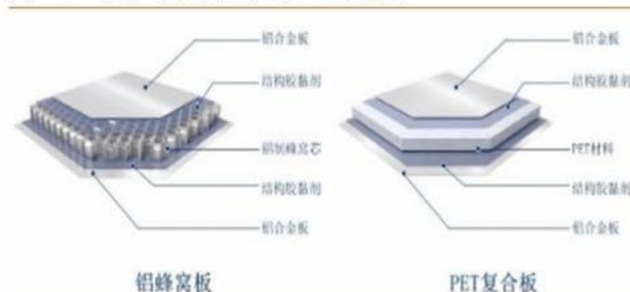
图 4：三明治复合材料内饰产品示意图
