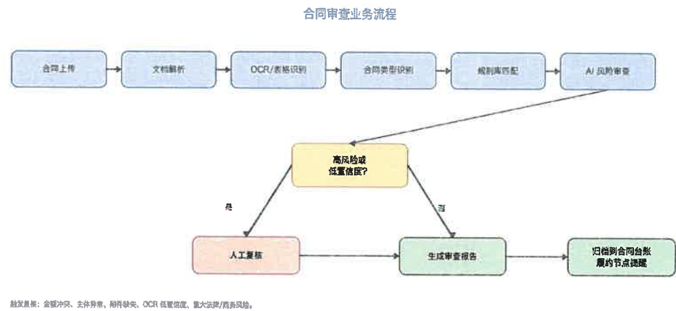
合同审查业务流程图
