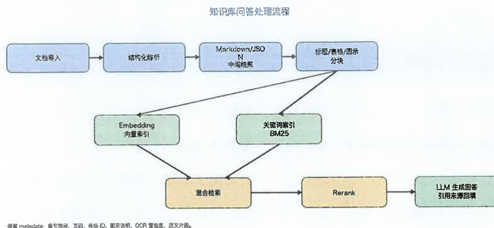
知识库问答处理流程图
