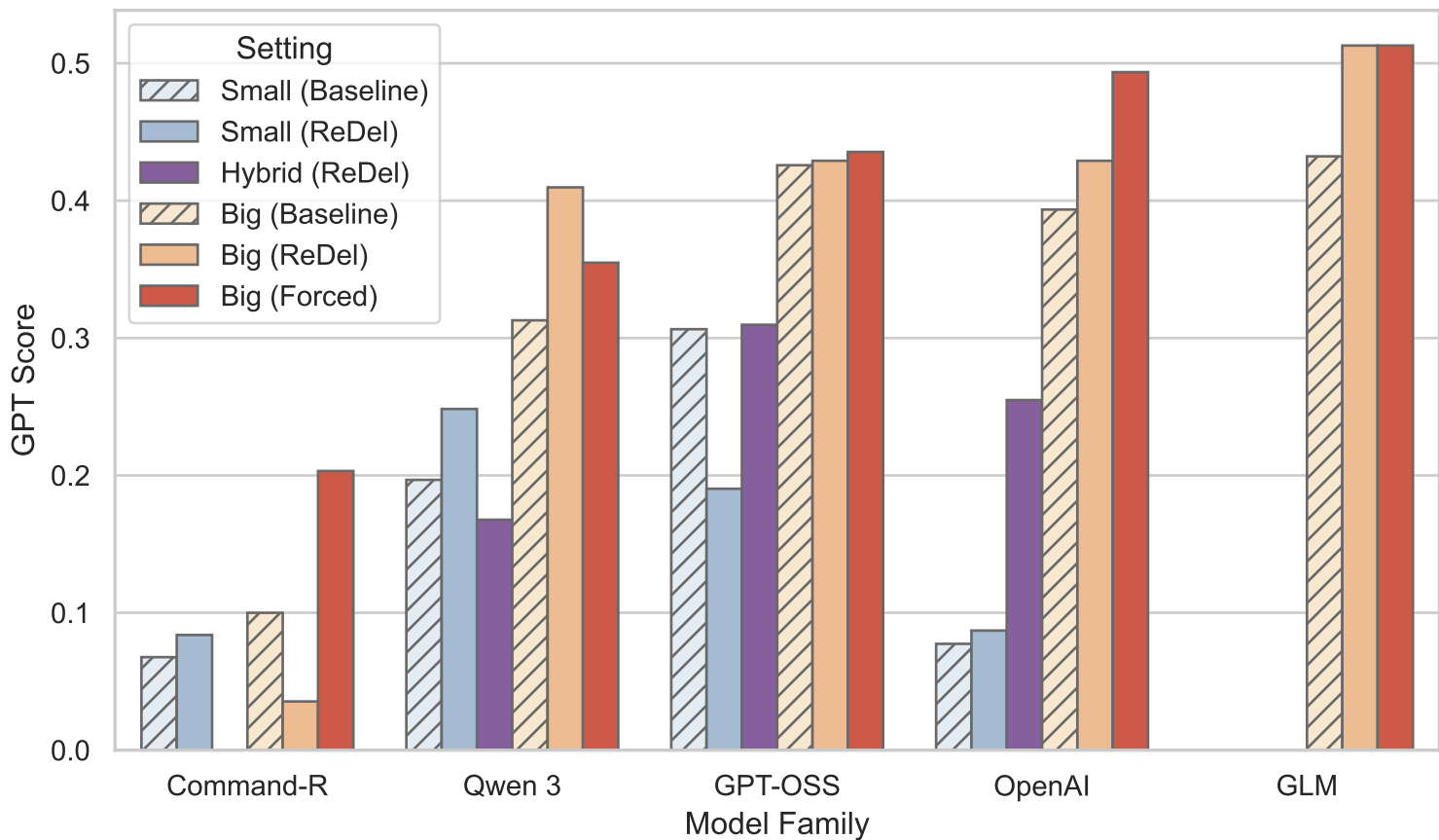
FanOutQA
