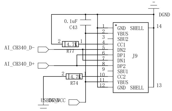
TYPE-C 单片机2烧录
