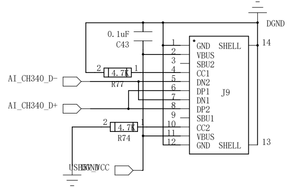
TYPE-C 单片机2烧录
