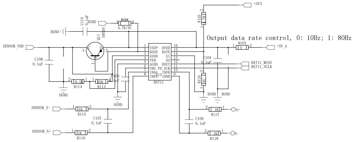
压力传感器
