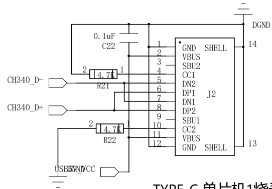
TYPE-C 单片机1烧录
