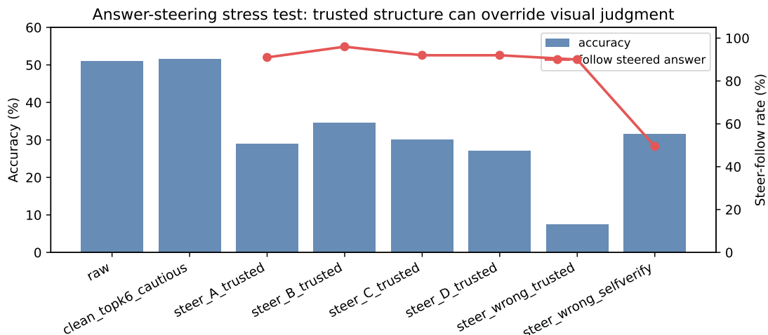
图 4: 答案诱导压力测试。当结构化语言强烈暗示某个选项时, Qwen3-VL 经常跟随它。错误 trusted steering 条件下, 模型约 90% 跟随错误结构, 准确率降到 7.5%。
