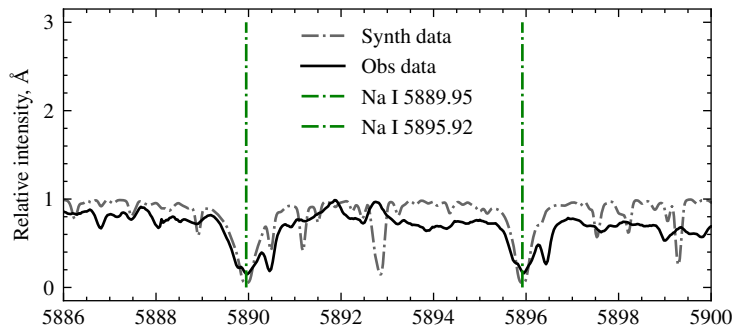
Na I line
