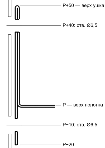
Сечение Г (поперёк полки, У 200), М 1:4: рёбра 8.2 — оси от наружной стенки бока
