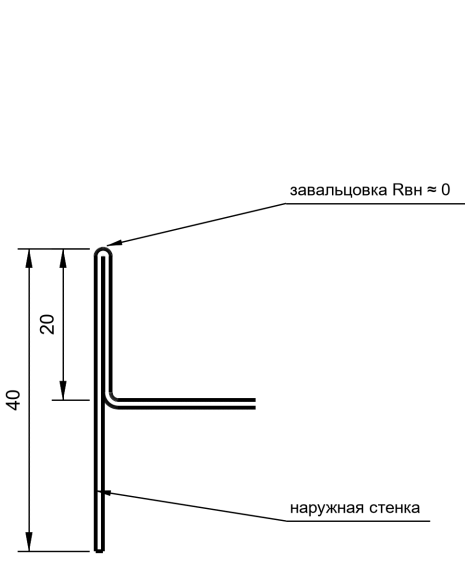
Сечение Г (поперёк полки, У 200), М 1:4: рёбра 8.2 — оси от наружной стенки бока
