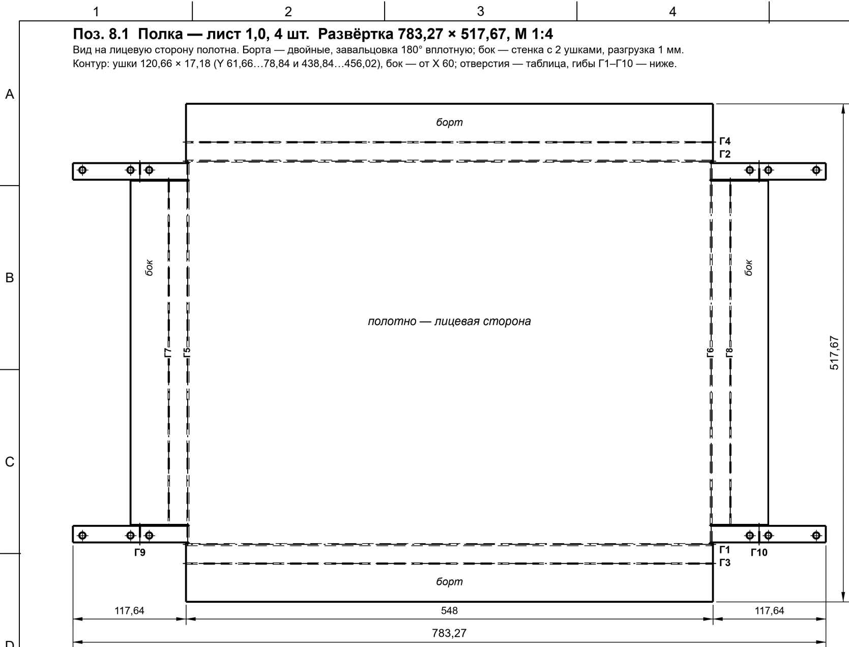
Отверстия поз. 8.1: 12 × Ø6,5, мм (от левого нижнего угла развёртки)
