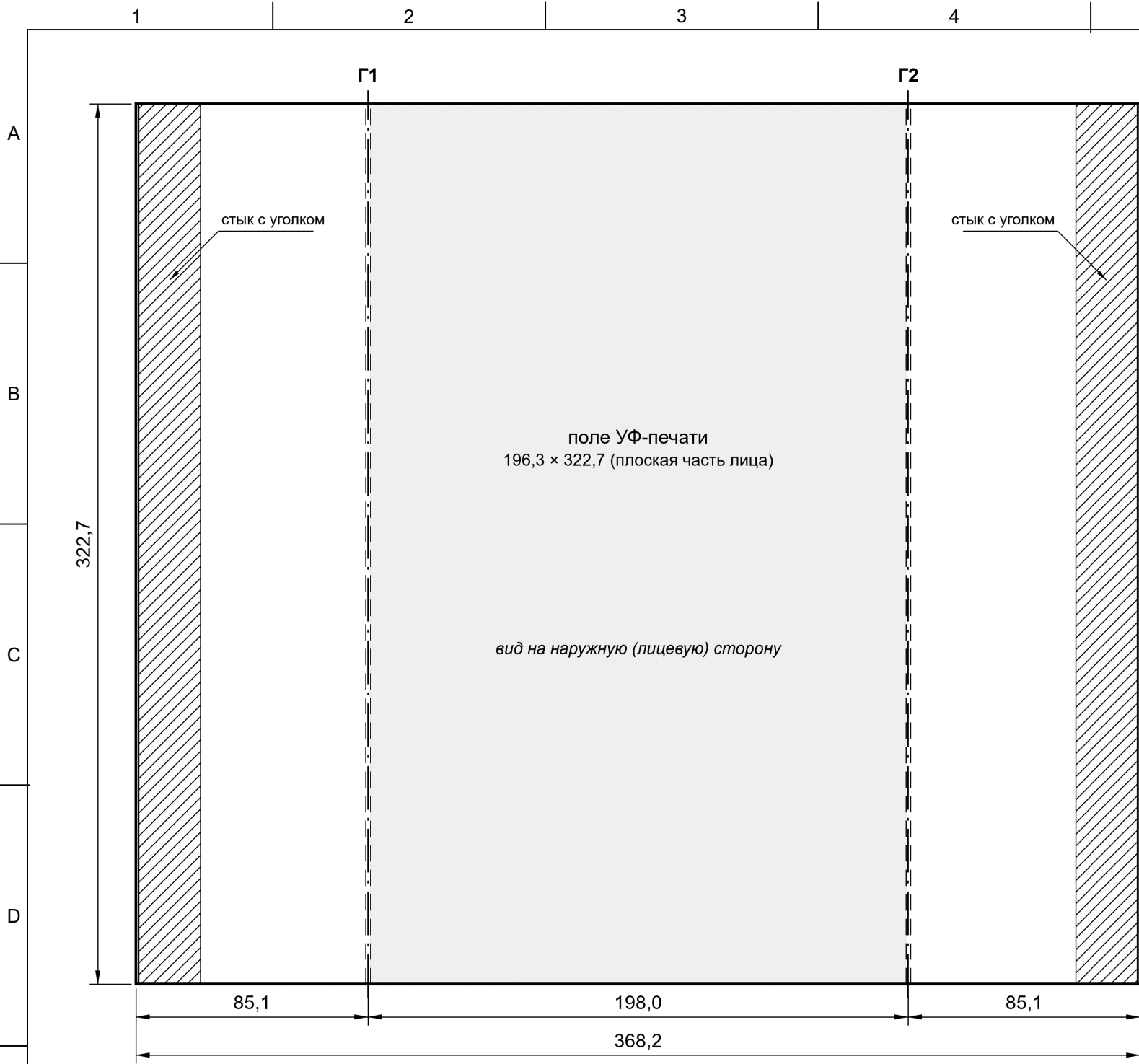
Поз. 1 Кожух — РЕТ/PVC 0,75, 1 шт. Развёртка 368,2 × 322,7, М 1:2
