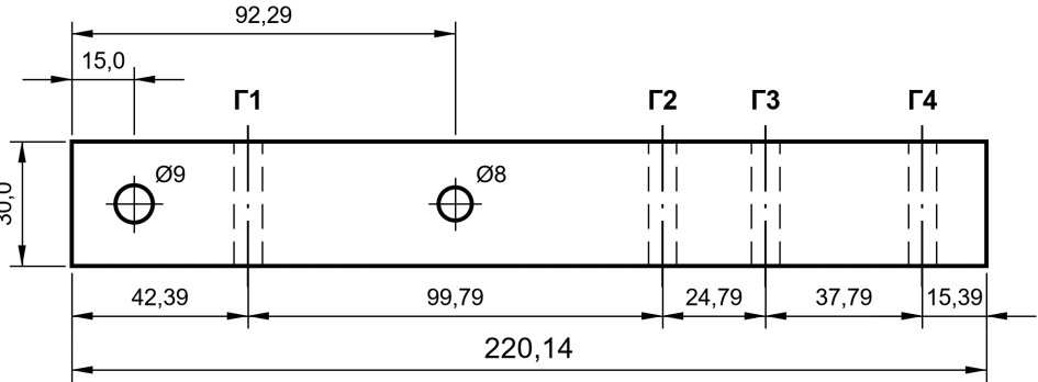
Поз. 5 Кронштейн задний — лист 3, 1 шт. Развёртка 220,1 × 30,0, М 1:2
