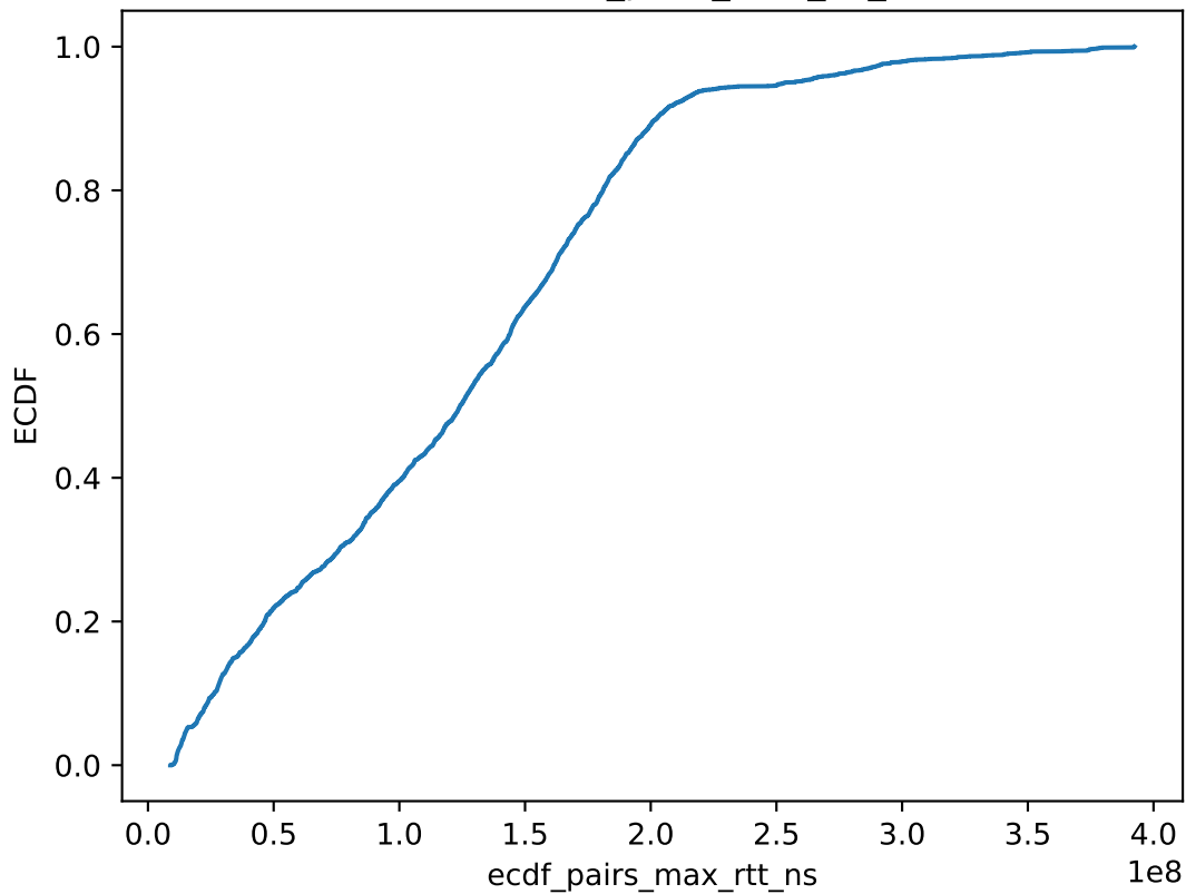
ECDF of ecdf_pairs_max_rtt_ns
