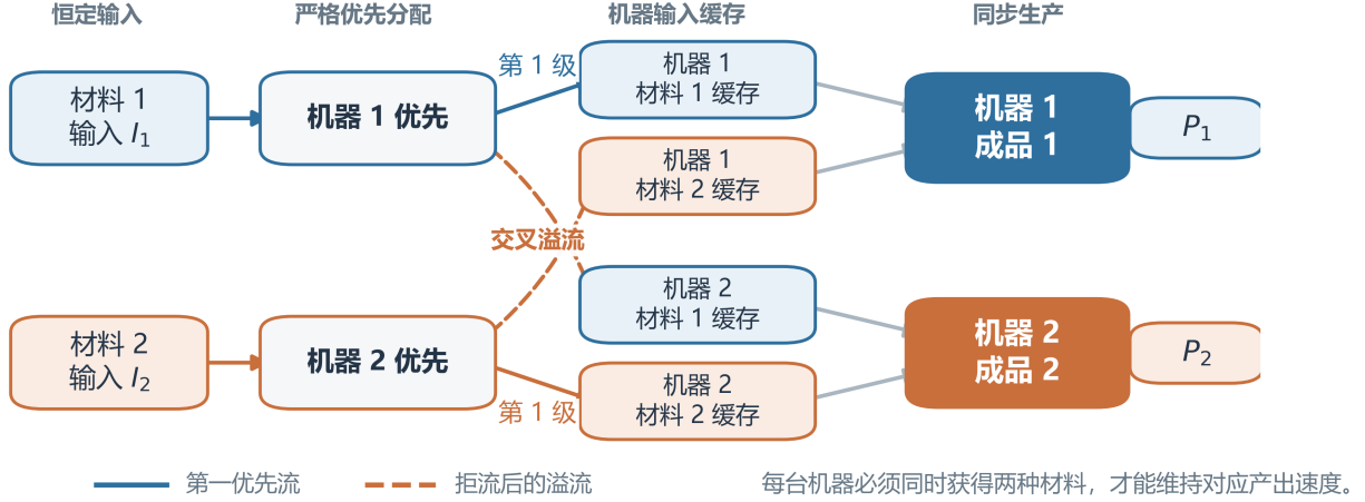
Figure 2: 两材料交叉严格优先供料拓扑。实线表示第一优先流，橙色虚线表示优先支路拒流后转向另一台机器的交叉溢流。
