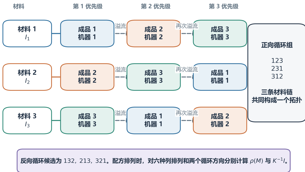
Figure 7: 三材料三级循环优先供料。三条材料链共同构成正向循环拓扑；相同颜色始终表示同一成品和机器。
