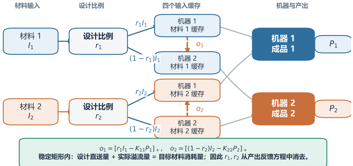
Figure 4: 设计比例分流与两条溢流补偿回路。设计比例只决定蓝色直送流量; 缓存拒流后产生的橙色溢流会改变实际分配。
