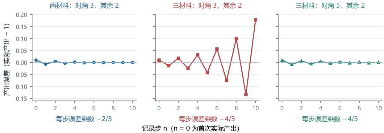
图 11: 两材料与三材料的共同产出误差。各图纵轴尺度相同，曲线表示每台机器相同的产出误差。对角系数为 3、其余系数为 2 时，两材料误差衰减，三材料误差交替放大；三材料的对角系数改为 5 后，误差重新衰减。右图改变了配方，不是仅调整原反例的优先级。
