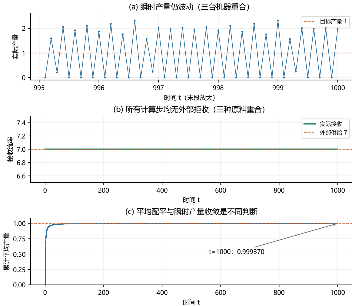
图 12: 空仓启动的三材料反例。上图放大末段的实际产量，三台机器曲线重合；中图给出原料实际接收流率；下图为从空仓起累计的平均产量。虚线标出目标产量或外部供给。有限时间波动与全量接收同时出现，不据此断言无限时间轨道必然振荡。
