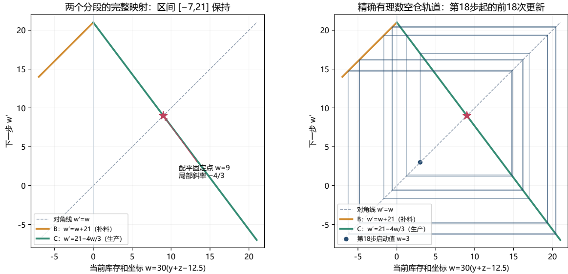
图 14: 归一化两分段映射及空仓早期轨道的蛛网图。橙段是斜率为 1 的停产补料，绿段是斜率为 -4/3 的生产更新，灰虚线为恒等映射。右图从精确启动值 w_{18} = 3 展示 18 次更新；图形帮助解释切换，长期结论依据正文证明。
