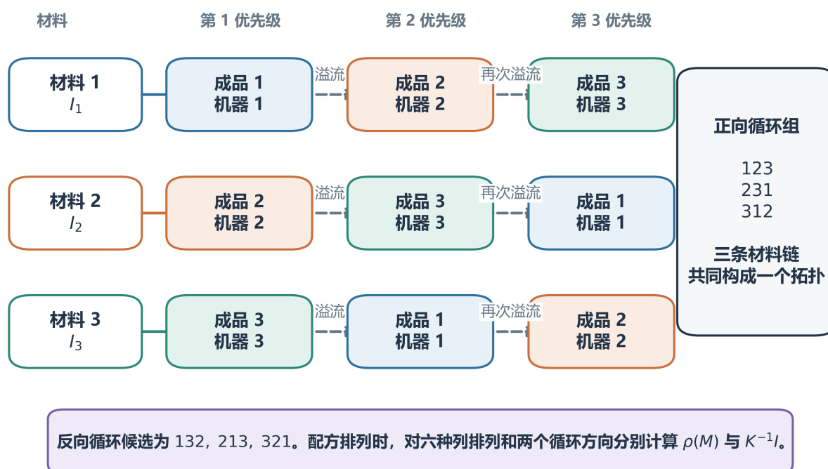
图 10: 三材料三级循环优先供料。三条材料链共同构成正向循环拓扑；相同颜色始终表示同一成品和机器。
