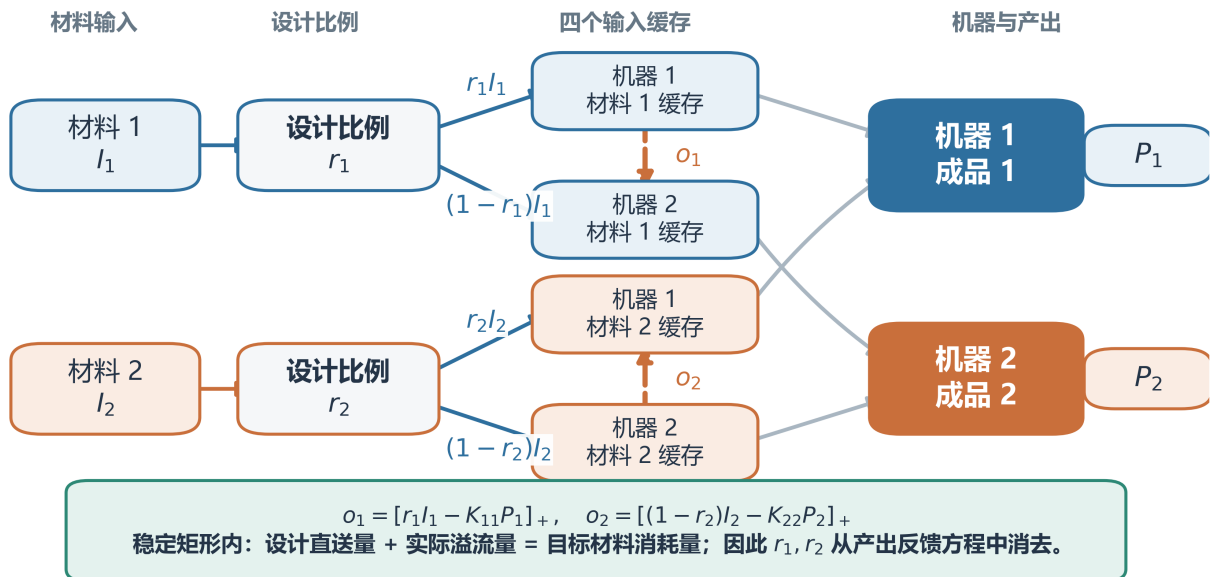
图 7: 设计比例分流与两条溢流补偿回路。设计比例只决定蓝色直送流量; 缓存拒流后产生的橙色溢流会改变实际分配。
