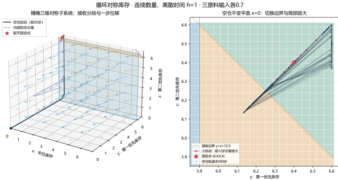
图 13: 循环对称子空间的三维分段相图及空仓不变平面。左图显示接收边界与一步位移；右图放大 x = 0 平面，橙线 y + z = 12.5 区分停产补料与末位到料生产。红星为配平点，红色小扰动显示局部交替放大。
