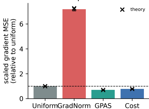
16-sample estimator
