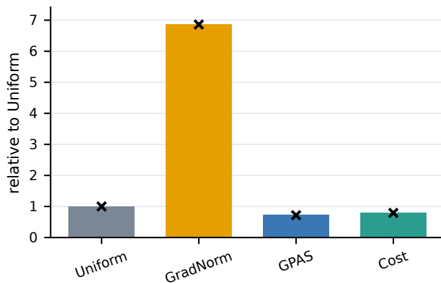
AdamW-metric estimator error
