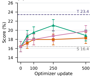
(d) LiveCodeBench v6
